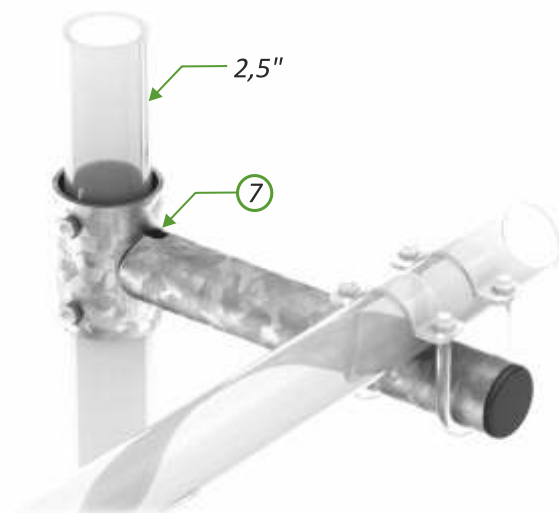
Łącznik DP regulowany
